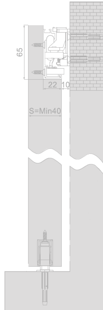
Embutida
