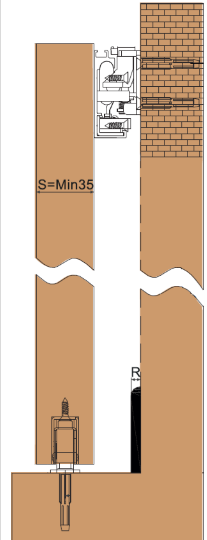
Sobreposta
